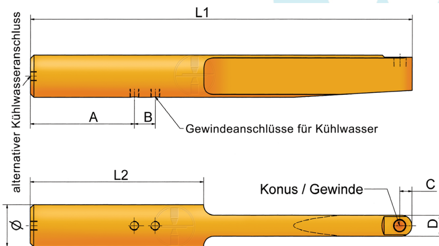
Abb. 5 Schwert-Arm
